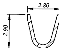
剖面 A-A 比例 5:1
